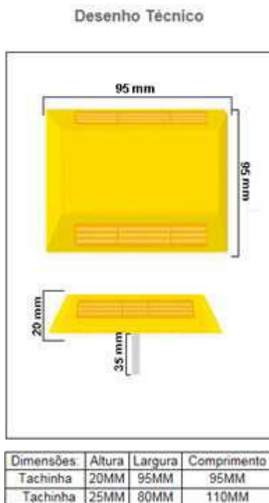
Figura A2 – Tachinha e Mini Tachão (95mmx95mm), Refletivo com Pino de Fixação
