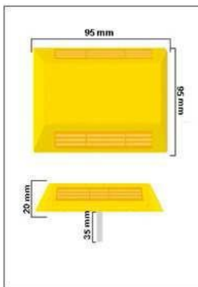
Desenho Técnico
