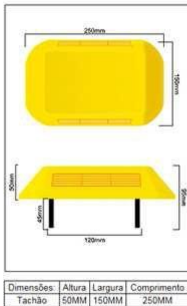
Figura A1 – Tachão Refletivo com Pino de Fixação
