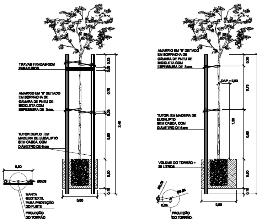
Figura 6: Tutoros simples e duplos.
