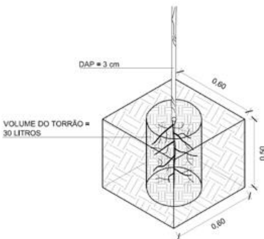
Figura 4: Dimensões da cova.
